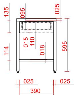
ELEVAÇÃO FRONTAL
